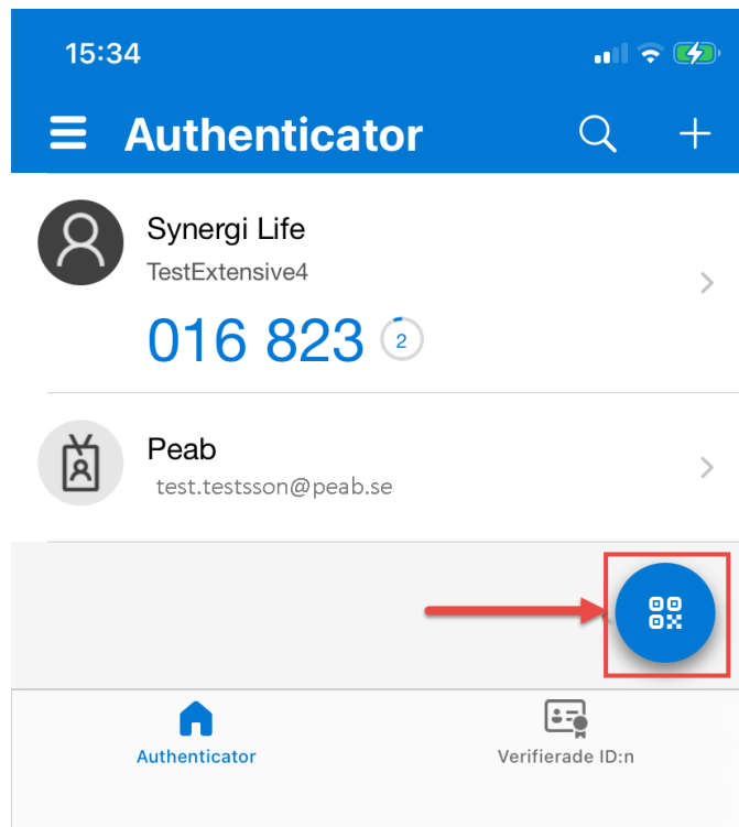
Bild 6. Authenticator konto
